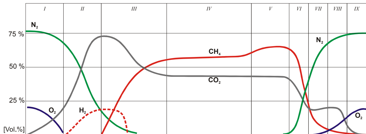
Abbildung 2 Verlauf der Deponiegaszusammensetzung in Abhängigkeit von der Zeit (Farquhar/Rovers 1973) mit Langzeitmodell Franzius 1981 sowie Rettenberger & Mezger 1992
